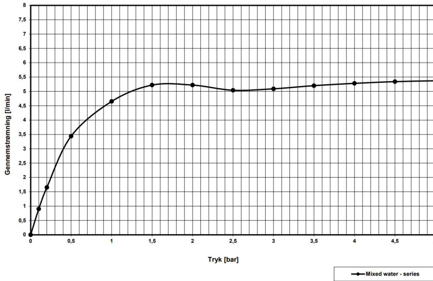
Flow diagram med spareperlator 5 l/min.
